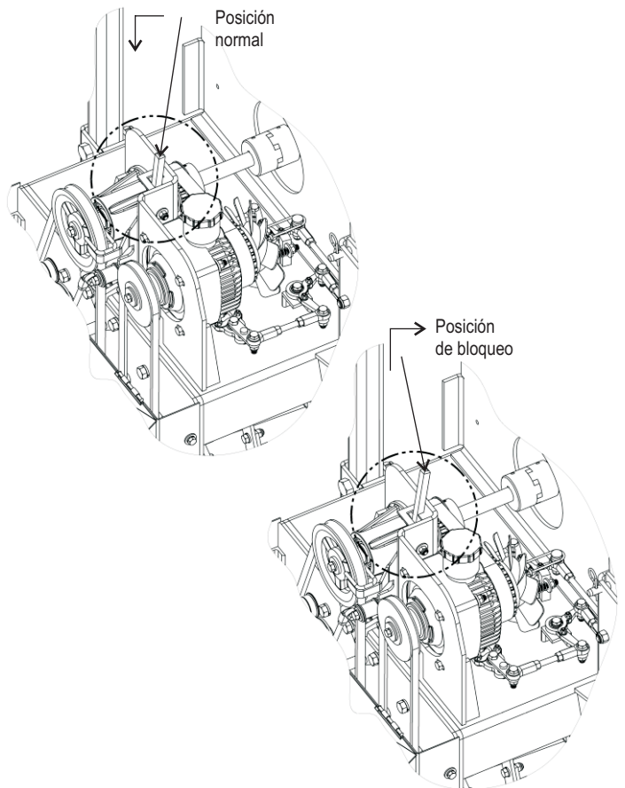
Figura 4. Palanca de la unidad hidrostática
