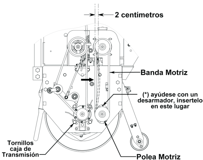
Figura 10. Banda motriz
