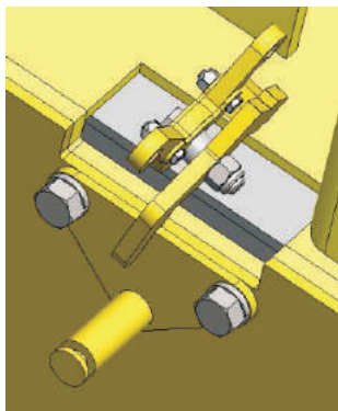
PIEZAS ENSAMBLADAS
