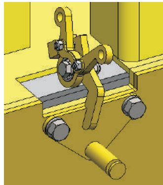
PIEZAS ENSAMBLADAS
